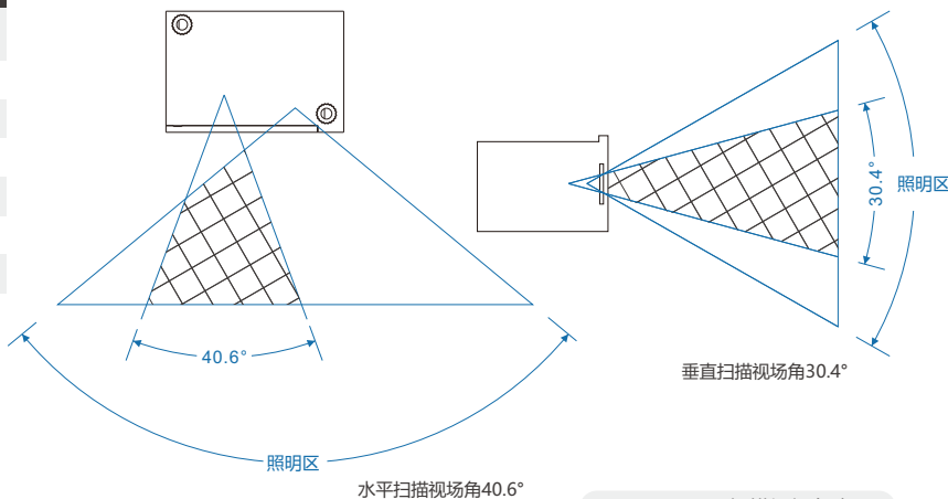
XL-3020GSQ扫描视场角度图
